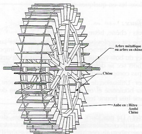
Roue construite au « Moulin du Parc » 27800 BOSROBERT
