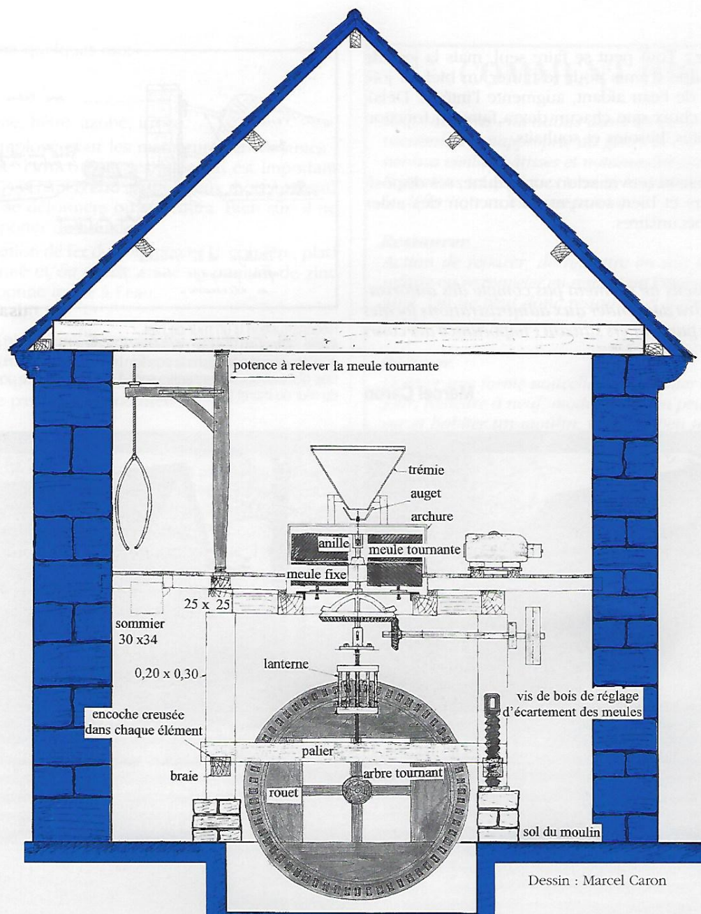
Coupe verticale du moulin du Parc en cours de réhabilitation 27800 Boisrobert
